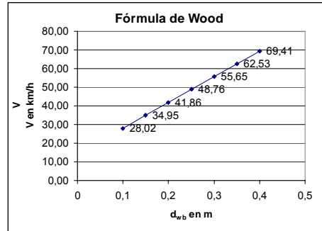
Gráfica No.2: velocidad de impacto vs deformación
